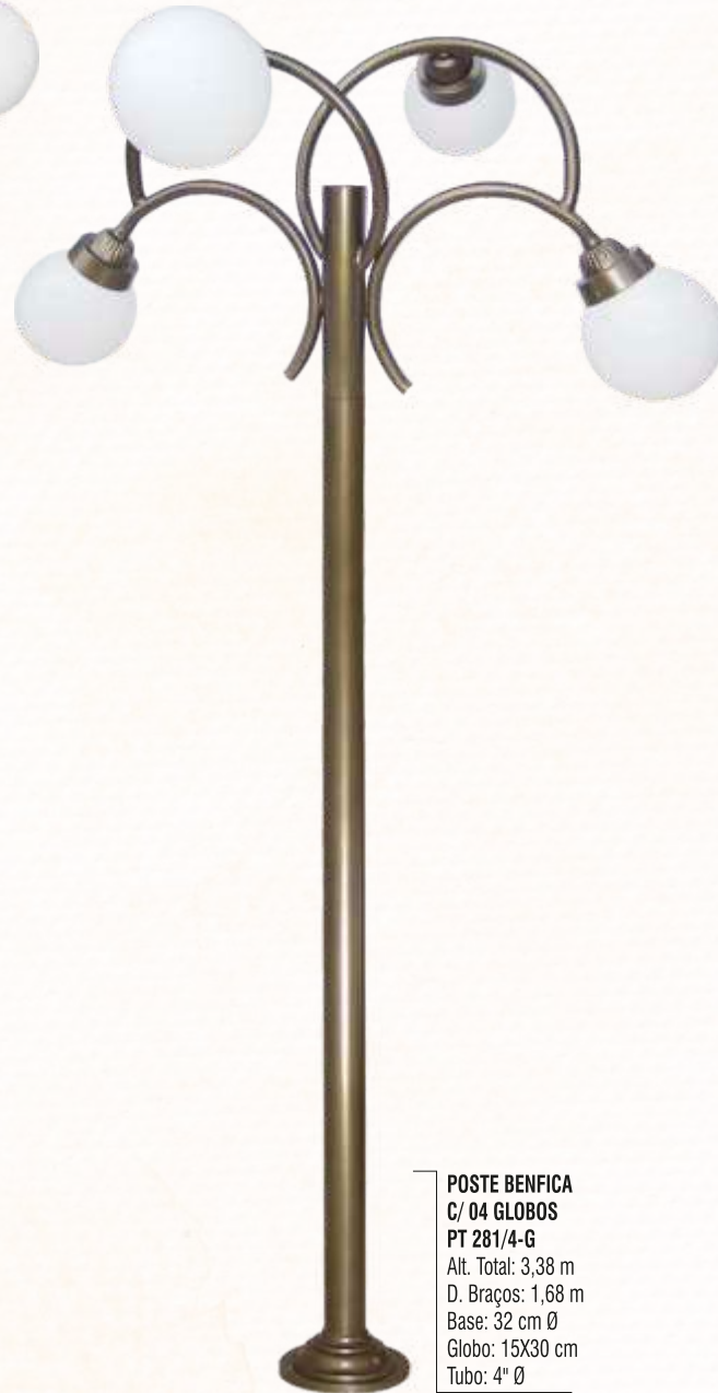
POSTE MONTREAL C/ 02 GLOBOS PT 288 / 2-G Alt. Total: 3,50 m D. Braços: 1,38 m Base: 32 cm Ø Globo: 15X30 cm Tubo: 4" Ø
