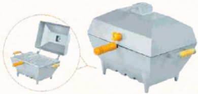
Churrasqueira a Bafo Quadrada Pequena Alt.: 28 cm - Larg.: 26 cm - Comp.: 43 cm
